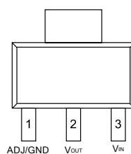
SOT-223-3L
